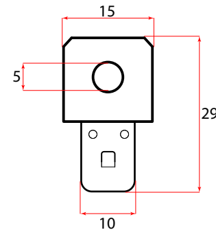
OPTIONAL BRACKET
